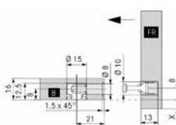
Front/bodem verbinding voor Scala
